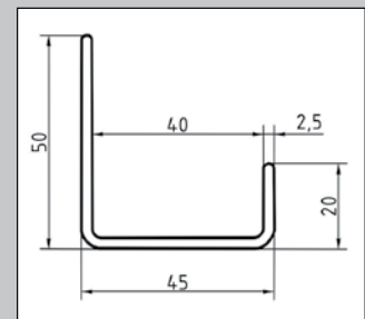
Rysunek dolnego profilu
