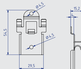
Klips fasadowy-Rhombus
